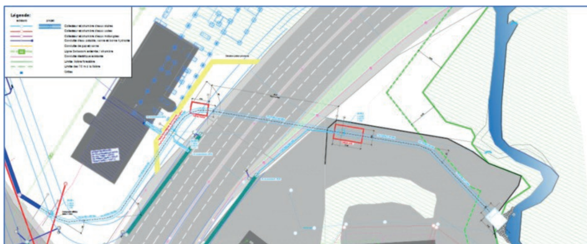
Tracé du collecteur Buyère Sorge
