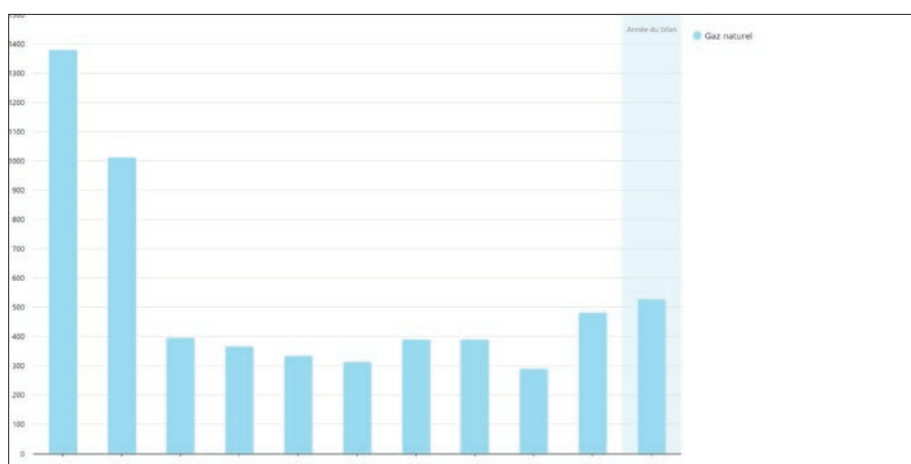
Graphique 7 : consommation d'énergie de chauffage (MWh) provenant du gaz
